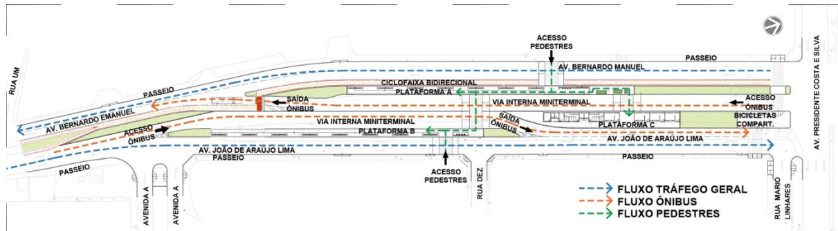
Figura 3 Implantação e planta de Fluxos
