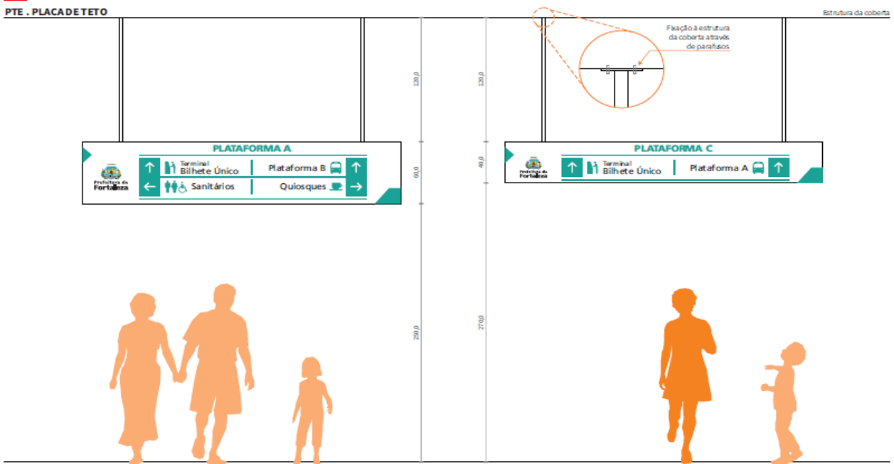
PTE Tipo 01 - Posicionamento medidas em centímetro Esc.: 1/20
