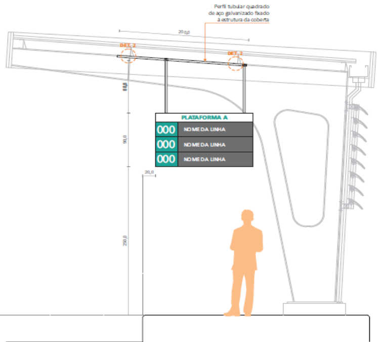
PTE Tipo 03 (Layout A) - Posicionamento medidas em centímetro Esc.: 1/25
