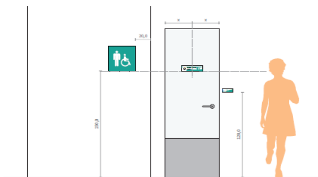
PPD / PBR / PPA - Posicionamento medidas em centímetro Esc.: 1/20
