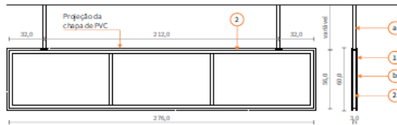
PTE Tipo 01 - Estrutura medidas em centímetro Esc.: 1/20
