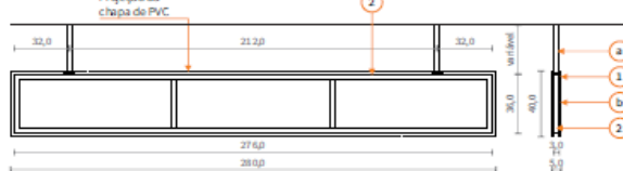
PTE Tipo 02 - Estrutura medidas em centímetro Esc.: 1/20
